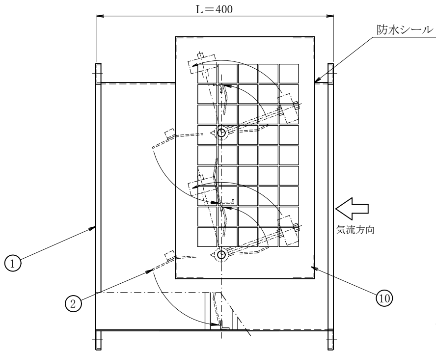
水平ダクト形 (羽根開放状態)
