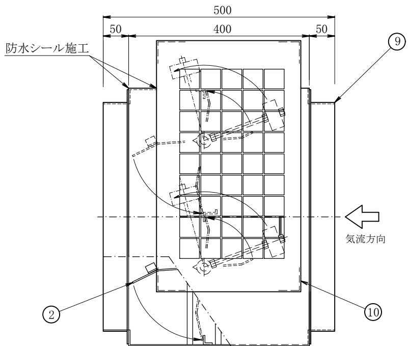
水平ダクト形 (羽根開放状態)
