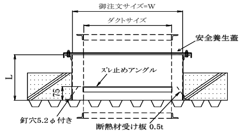
◎現地据付詳細
