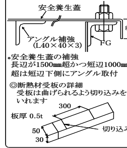
◎安全養生蓋(1.6t)の取付詳細
