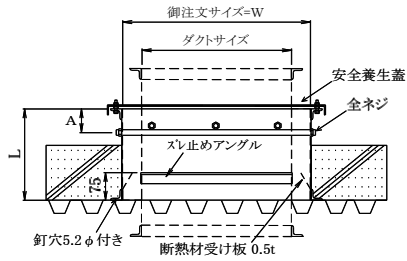
◎現地据付詳細
