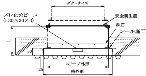
◎現地据付詳細
