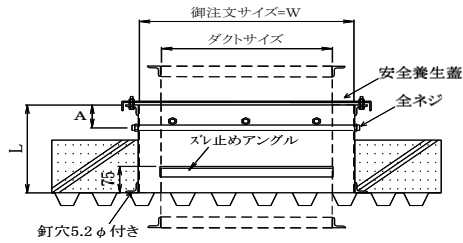
◎現地据付詳細
